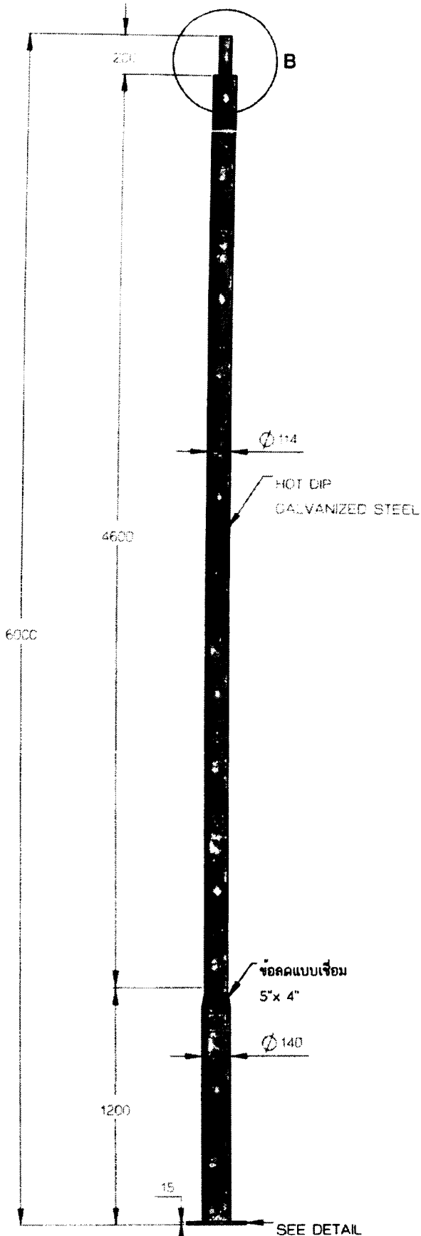
HI-WCS-060:เสากลมสูง6เมตรขนาด5นิ้วลด4นิ้ว SCALE 1 : 28
